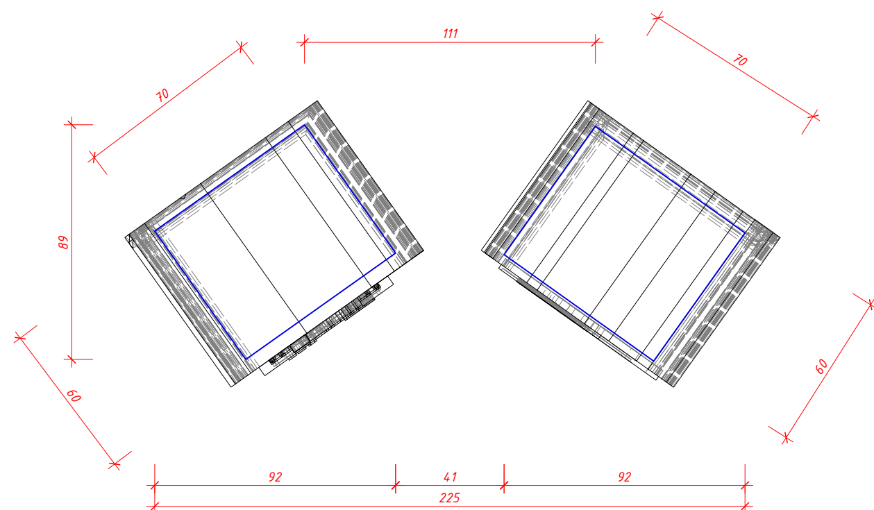
RZUT
