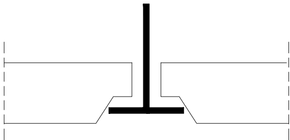
DETAL MODUŁOWEGO SUFITU PODWIESZANEGO O UKRYTEJ KRAWĘDZI
