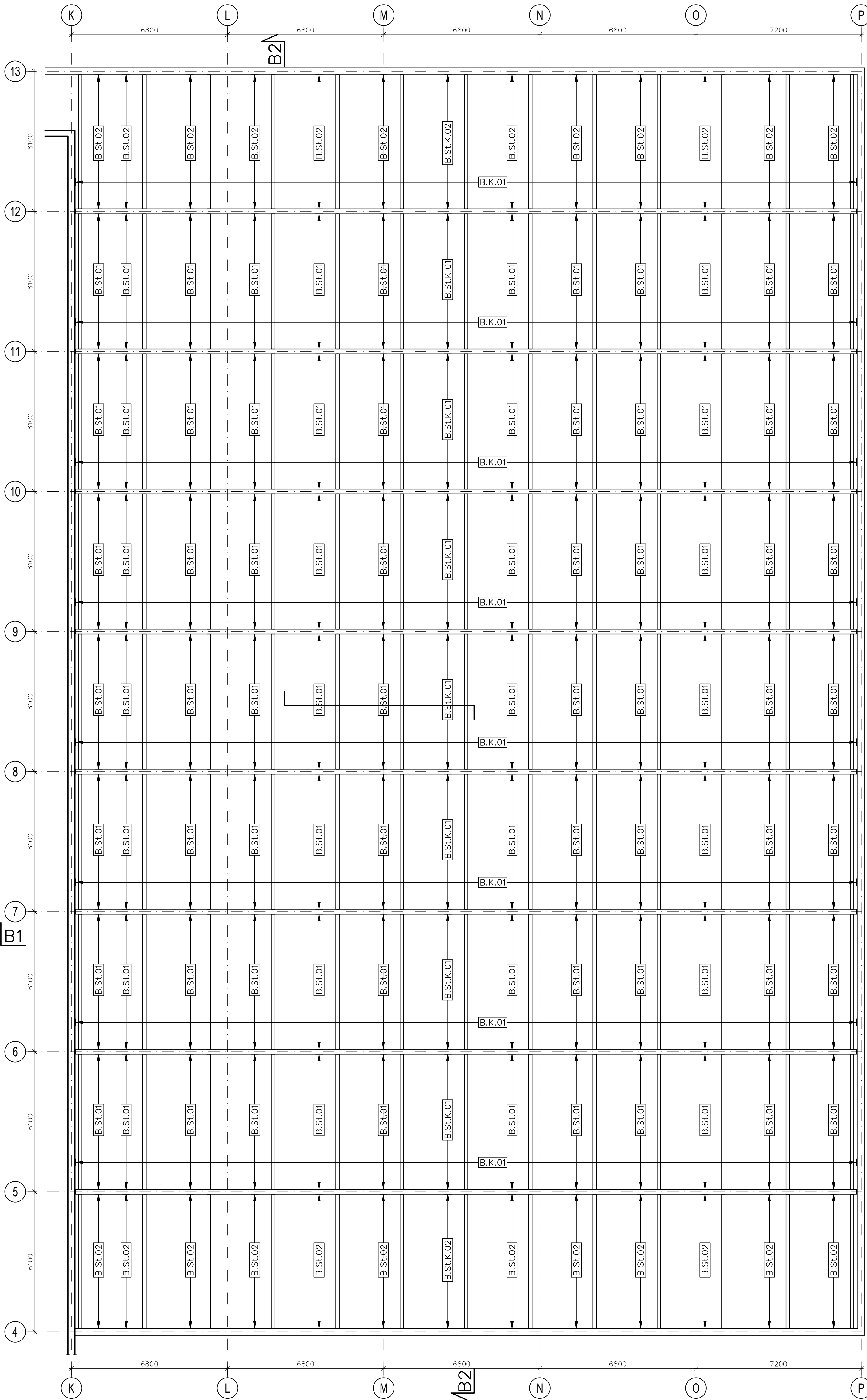
Schemat zadaszenia hali B
